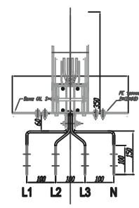
Разрез 'A' - 'A'
