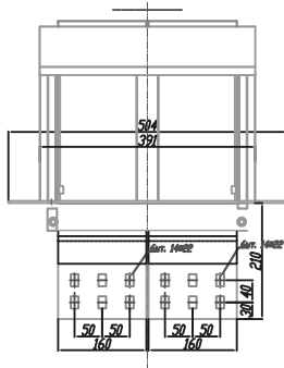
Разрез 'B' - 'B'
