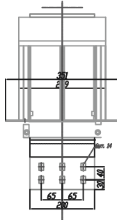
Разрез 'B' - 'B'
