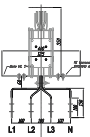
Разрез 'A' - 'A'
