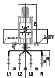
Разрез 'A' - 'A'
