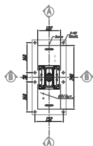
AL 630A Фланцевый блок 3P4W 100%N PE-корпус IP54
