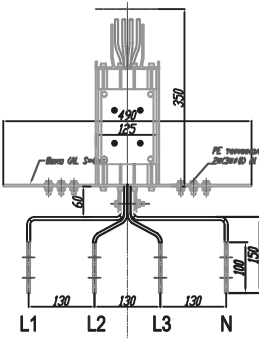
Разрез 'A' - 'A'
