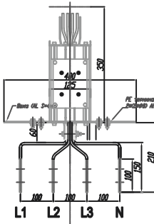
Разрез 'A' - 'A'
