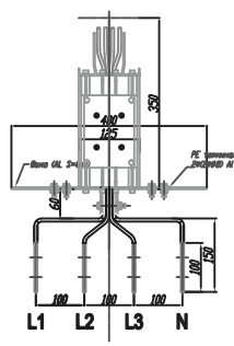
Разрез 'A' - 'A'
