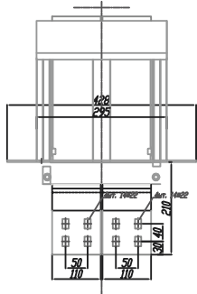
Разрез 'B' - 'B'
